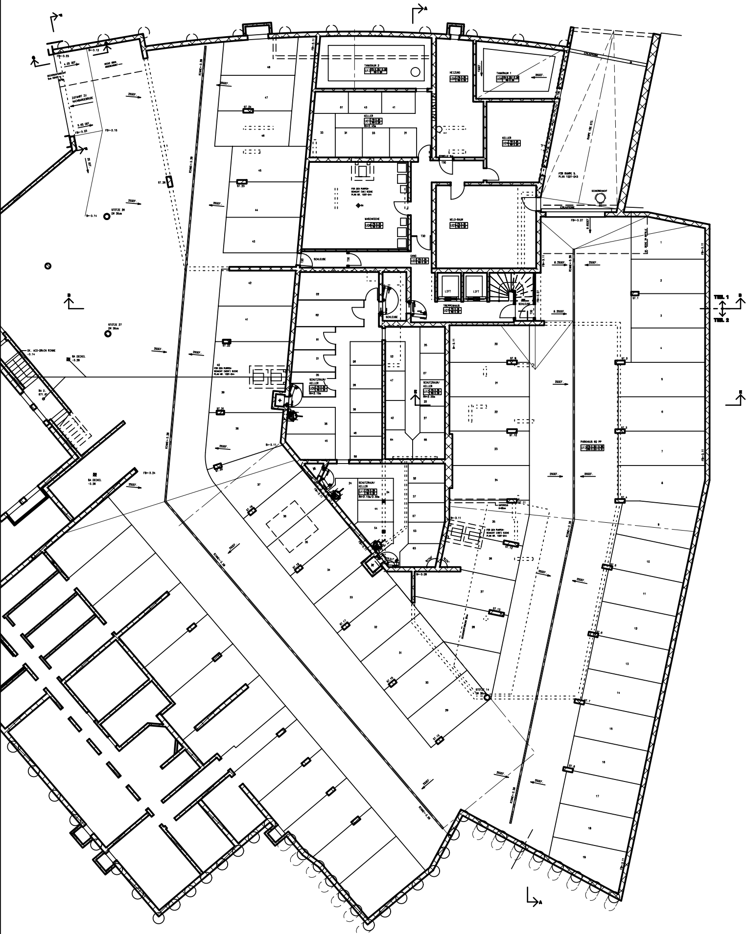
WOHNPAK VIKTORIA UNTERGESCHOSS 1:250 ARCHITEKTUR ATELIER BALZANI GMBH BRIG 30.10.2006
